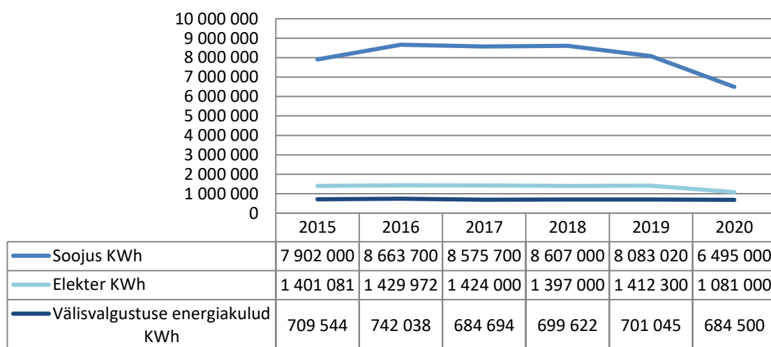
Joonis 1.1.14. Munitsipaalhoonete energiatarve ja välisvalgustuse energiakulud.
