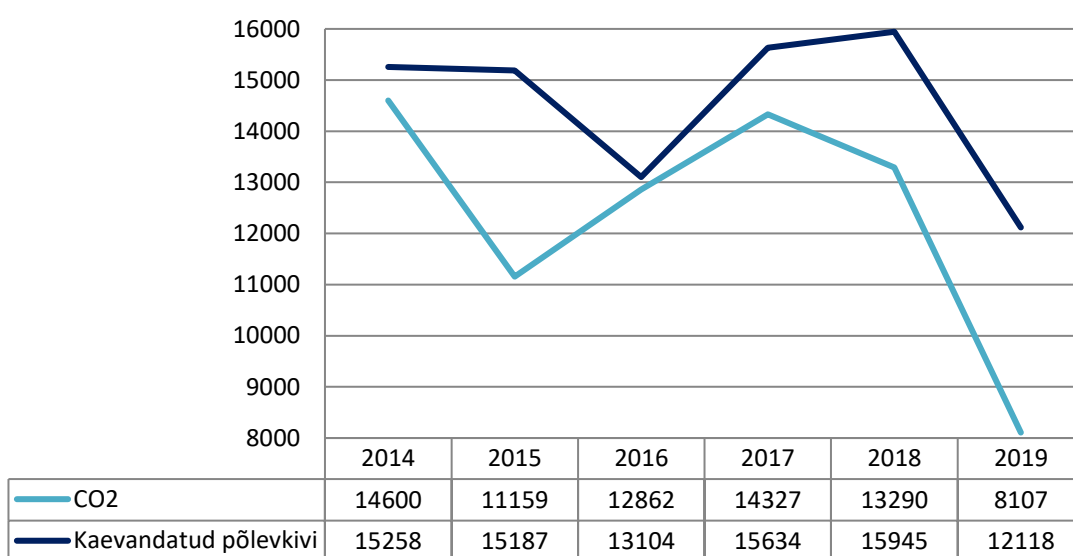
Joonis 1.1. 20. Põlevkivisektori kaasnevad õhuheitmed – CO 2 (tuh tonni). Allikas: Eesti põlevkivitööstuse aastaraamat
