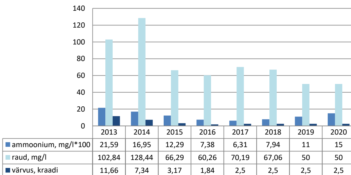
Joonis 1.1.19. Joogivee keskmised näitajad 5 . Allikas: Sillamäe Veevärk
