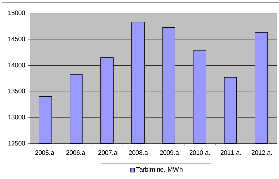
Joonis 3.27. Elanike elektritarbimine läbi VKG Elektrivõrgud OÜ
