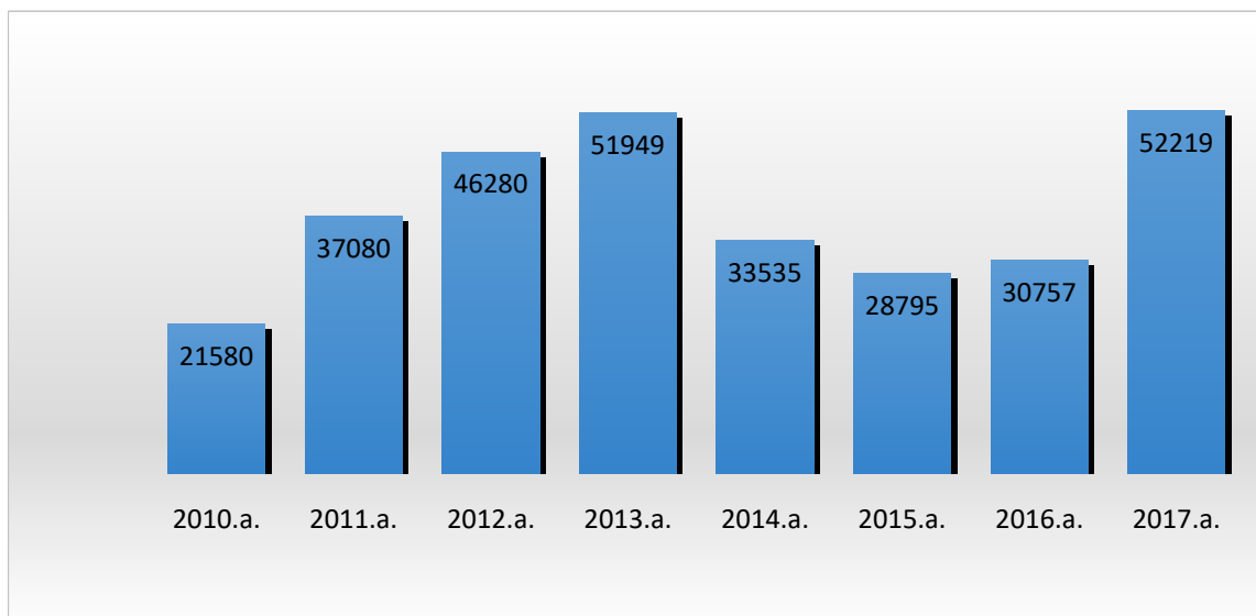
Joonis 28. Asutuste elektritarbimine (MWh) läbi VKG Elektrivõrgud OÜ
