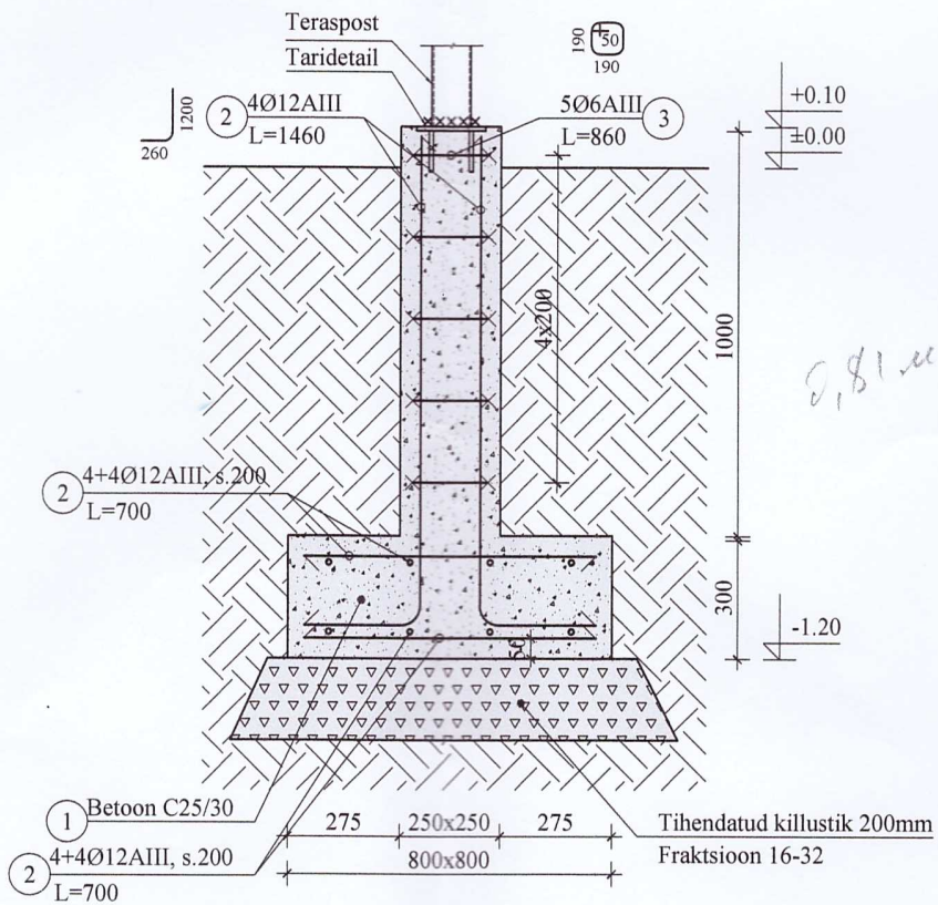
a-a M 1:20
